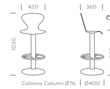
Colonna Column Ø76 | Ø400 Meccanismo di ritorno automatico Automatic return mechanism
